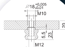
拉栓孔位加工圖
